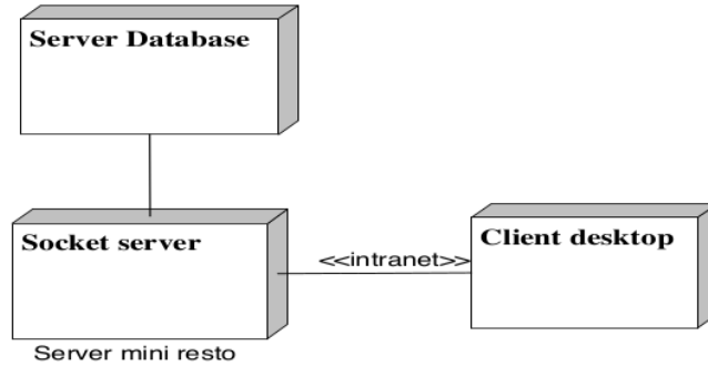
Gambar 4. Deployment Diagram Sistem Pemesanan Di Mini Resto
