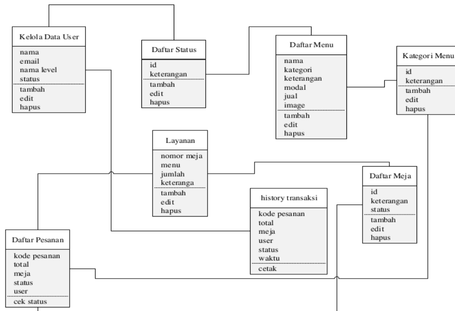
Gambar 2. Class Diagram Sistem Pemesanan Pada Mini Resto
