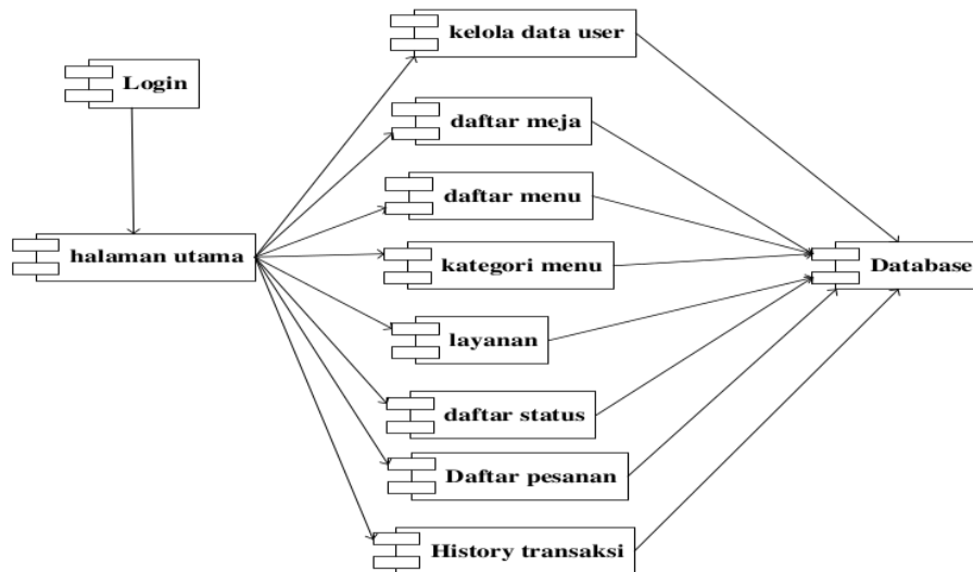
Gambar 3. Component Diagram Sistem Pemesanan Pada Mini Resto
